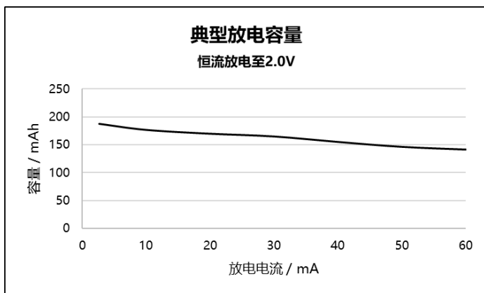
典型放电曲线
